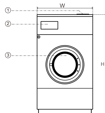
正视图 FRONT
