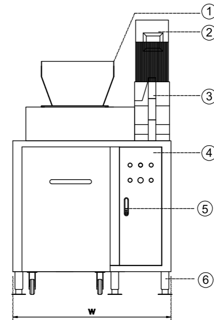
正视图 FRONT
