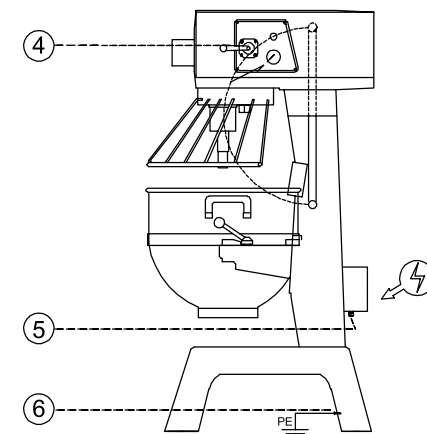
右视图 RIGHT
