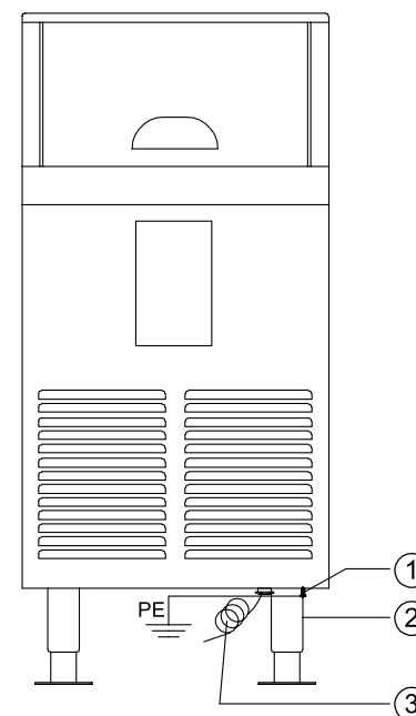
正视图 FRONT
