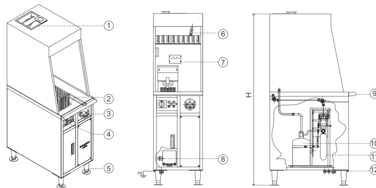
示意图 DIAGRAMMATIC
